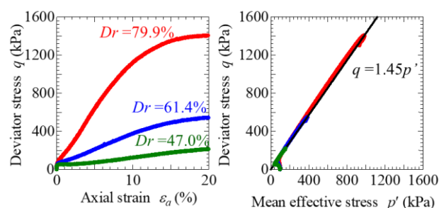
図8 細粒分10%流出試料の非排水三軸試験結果
