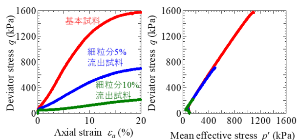
図5 細粒分の流出による非排水せん断挙動の変化
