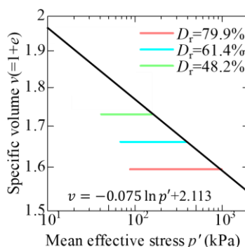
図 12 細粒分 10%流出試料の限界状態線
