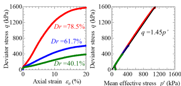
図6 基本試料の非排水三軸試験結果
