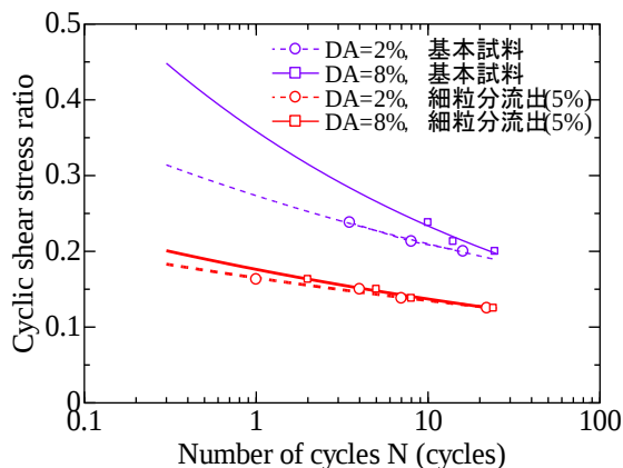
図 17 細粒分流出による液状化強度曲線の違い
