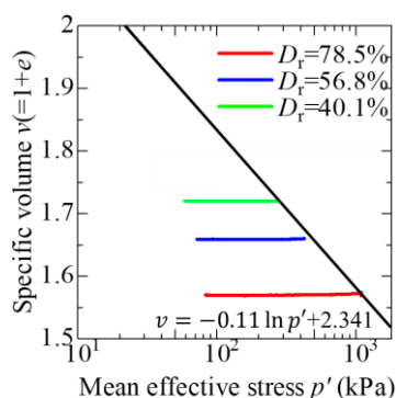
図 10 基本試料の限界状態線
