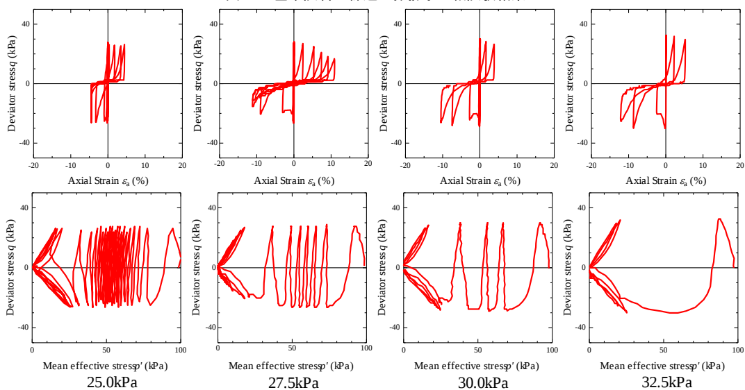
図 14 細粒分 5%流出試料の繰返し非排水三軸試験結果
