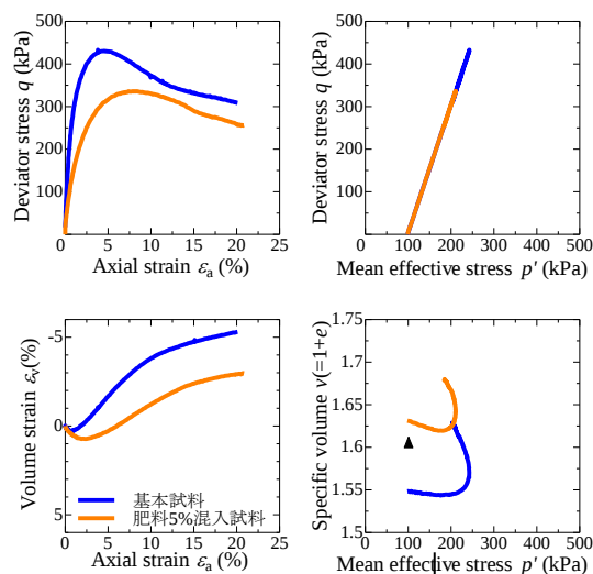
図 3 基本試料と肥料 5%混入試料の比較
