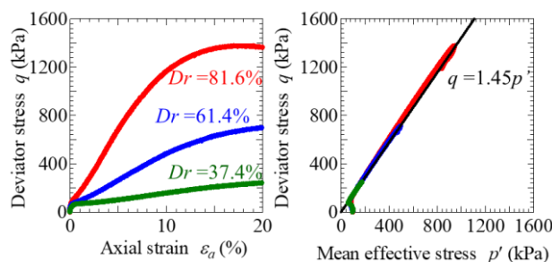
図7 細粒分5%流出試料の非排水三軸試験結果
