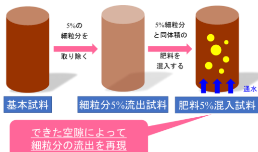
図2 肥料を用いた細粒分の流出の模擬方法
