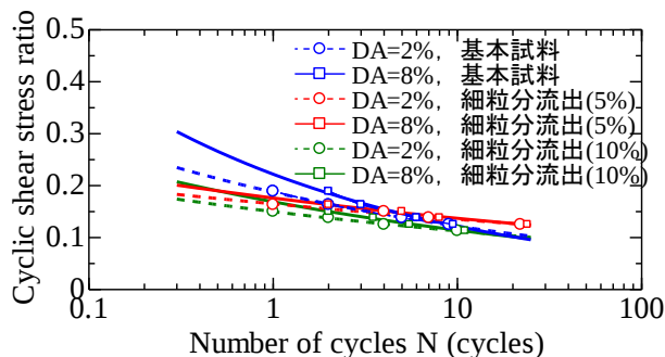
図 16 粒度の違いによる液状化強度曲線の違い
