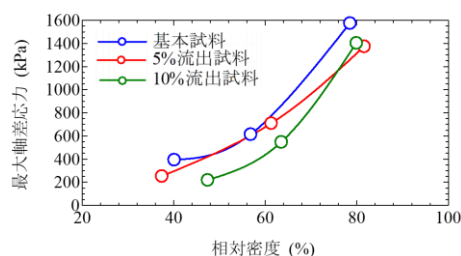
図9 最大軸差応力と相対密度の関係
