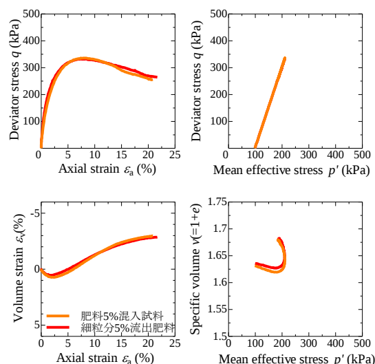
図 4 肥料 5%混入試料と細粒分 5%流出試料の比較
