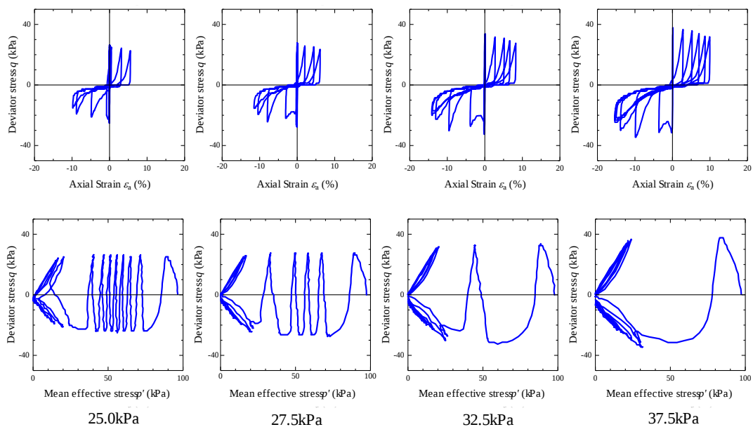
図 13 基本試料の繰返し非排水三軸試験結果
