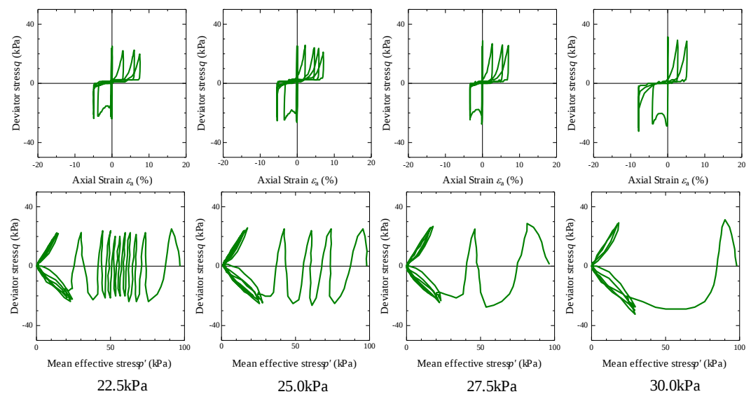
図 15 細粒分 10%流出試料の繰返し非排水三軸試験結果
