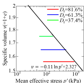
図 11 細粒分 5%流出試料の限界状態線
