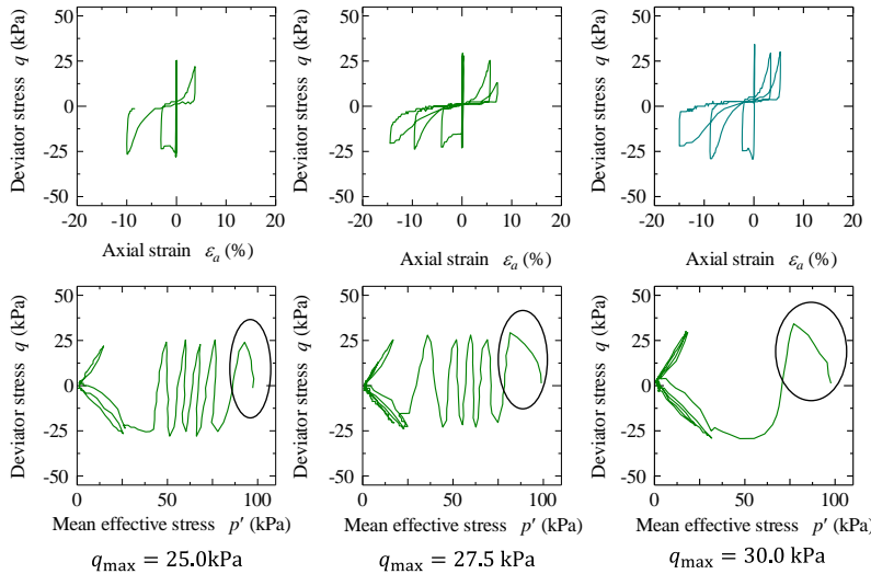
図-6 肥料混入試料の非排水繰返しせん断試験結果
