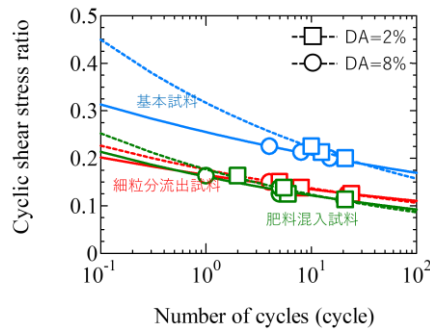
図-7 液状化強度曲線の比較
