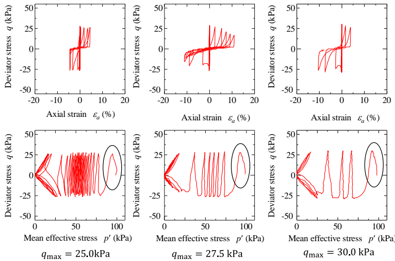
図-5 細粒分流出試料の非排水繰返しせん断試験結果
